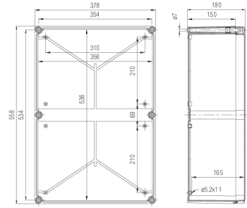
SOLID 558x378x180
